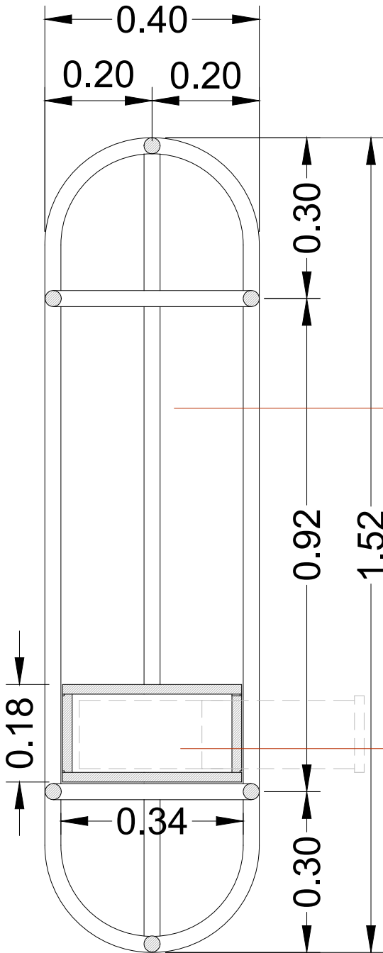
CORTE 1-1
