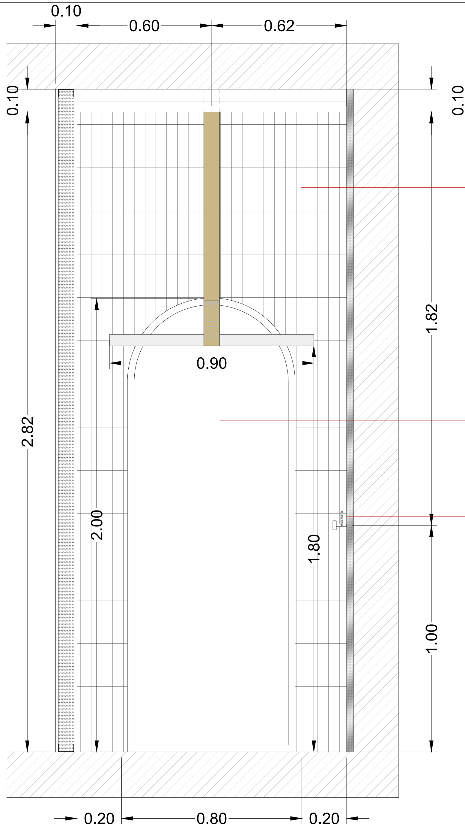
CORTE A-A
