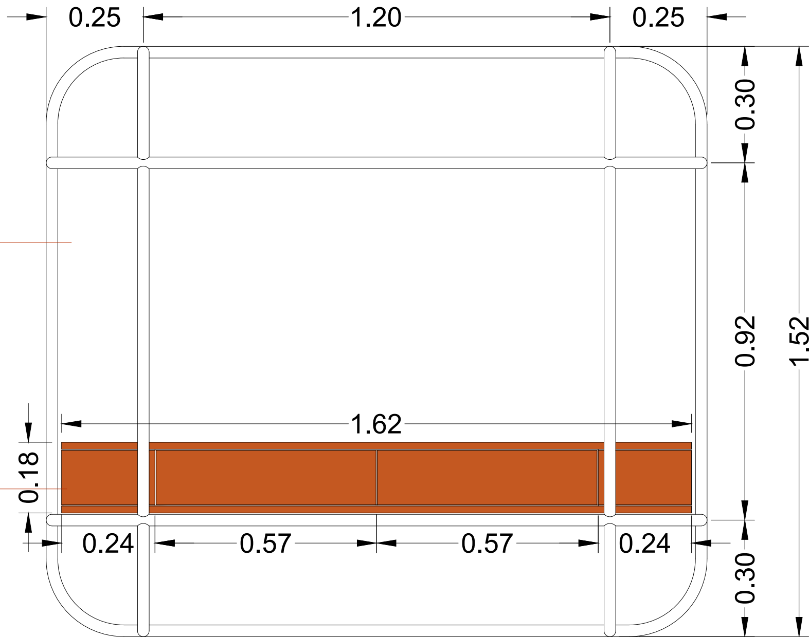
VISTA
