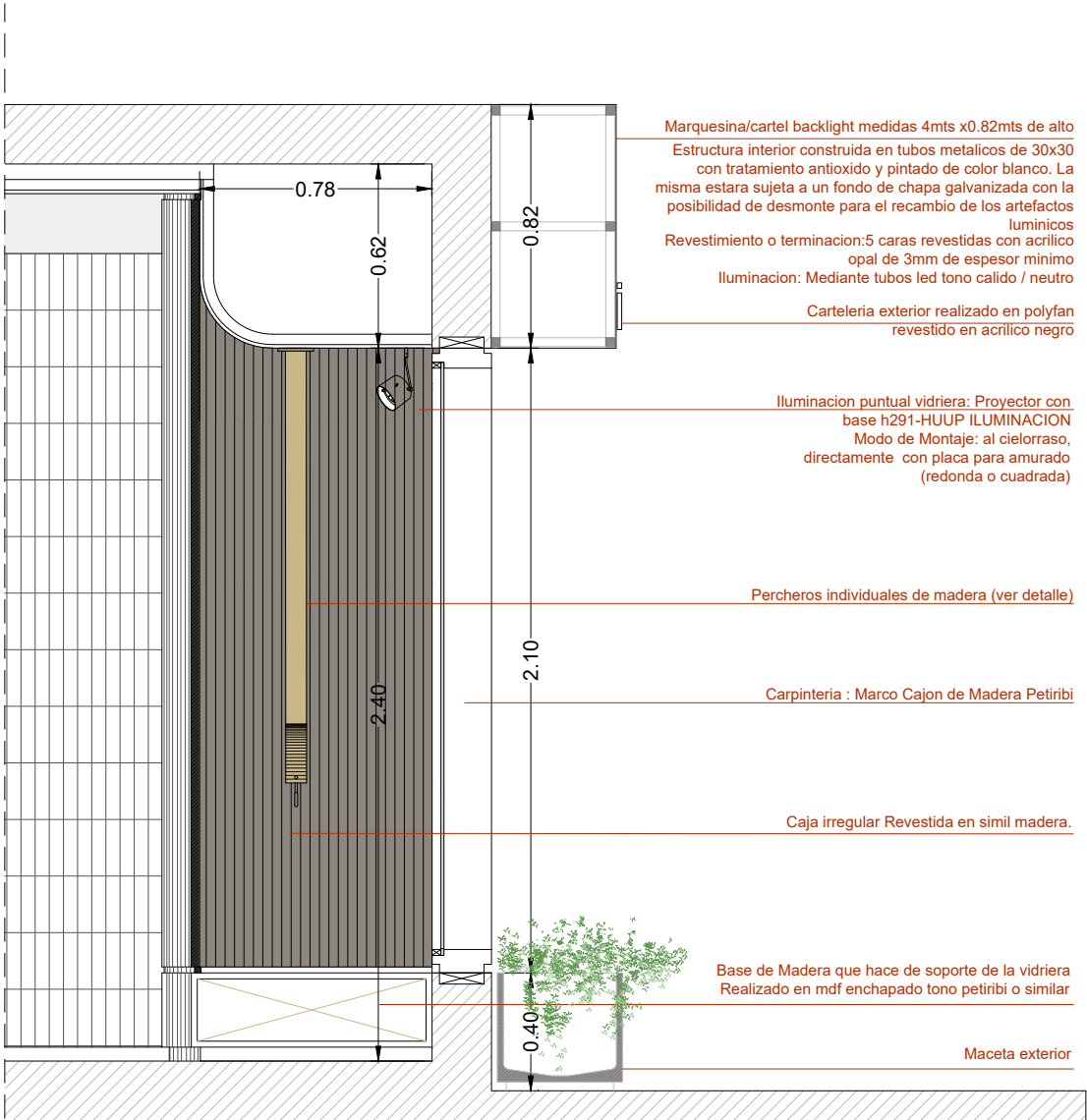
CORTE 3-3 1:25
